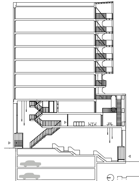
Doorsnedes 1:500
