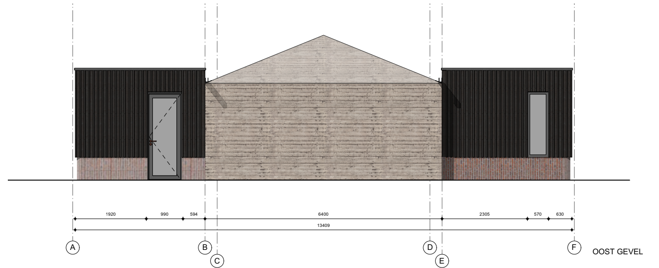
GEVELS NIEUWE SITUATIE BIJGEBOUW BUNKER
