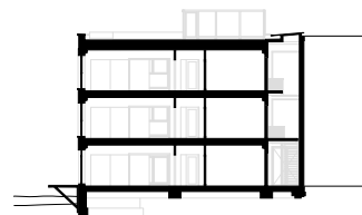
Dwarsdoorsnede deelschool
