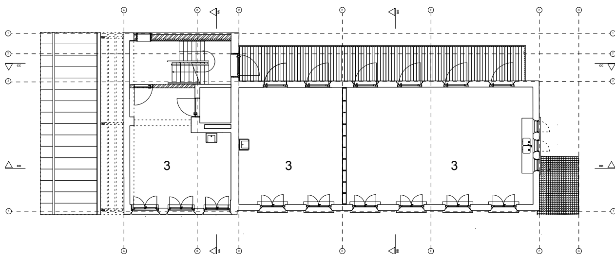
Niveau +1 (jeugdlokalen)
