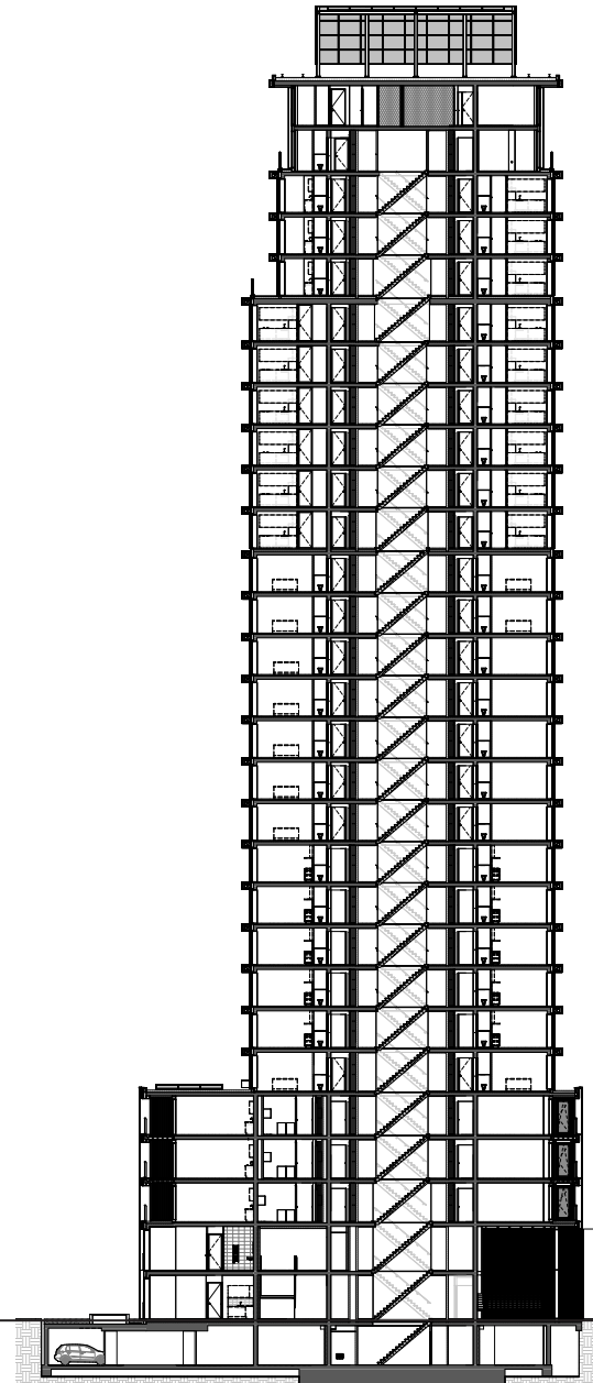
Doorsnede A-A, 1:600
