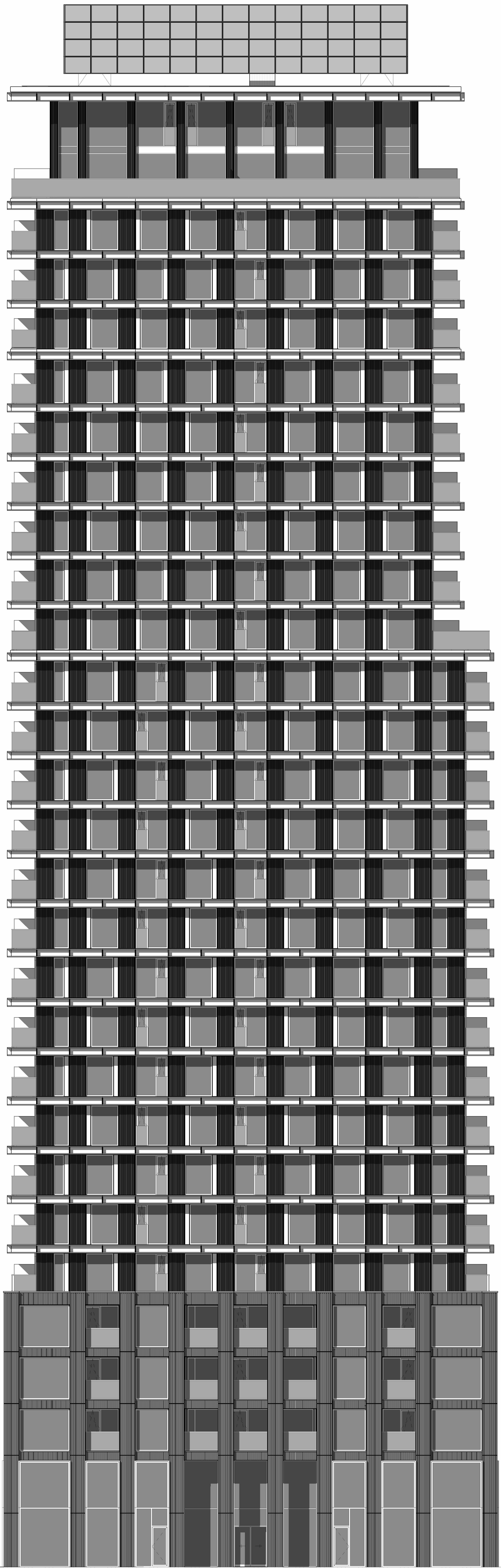
Noordgevel, 1:100
