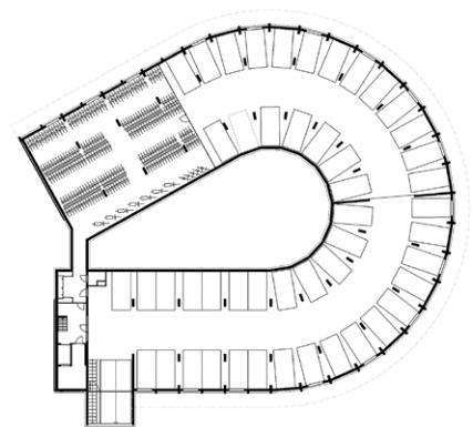
Halfverdiepte kelder
