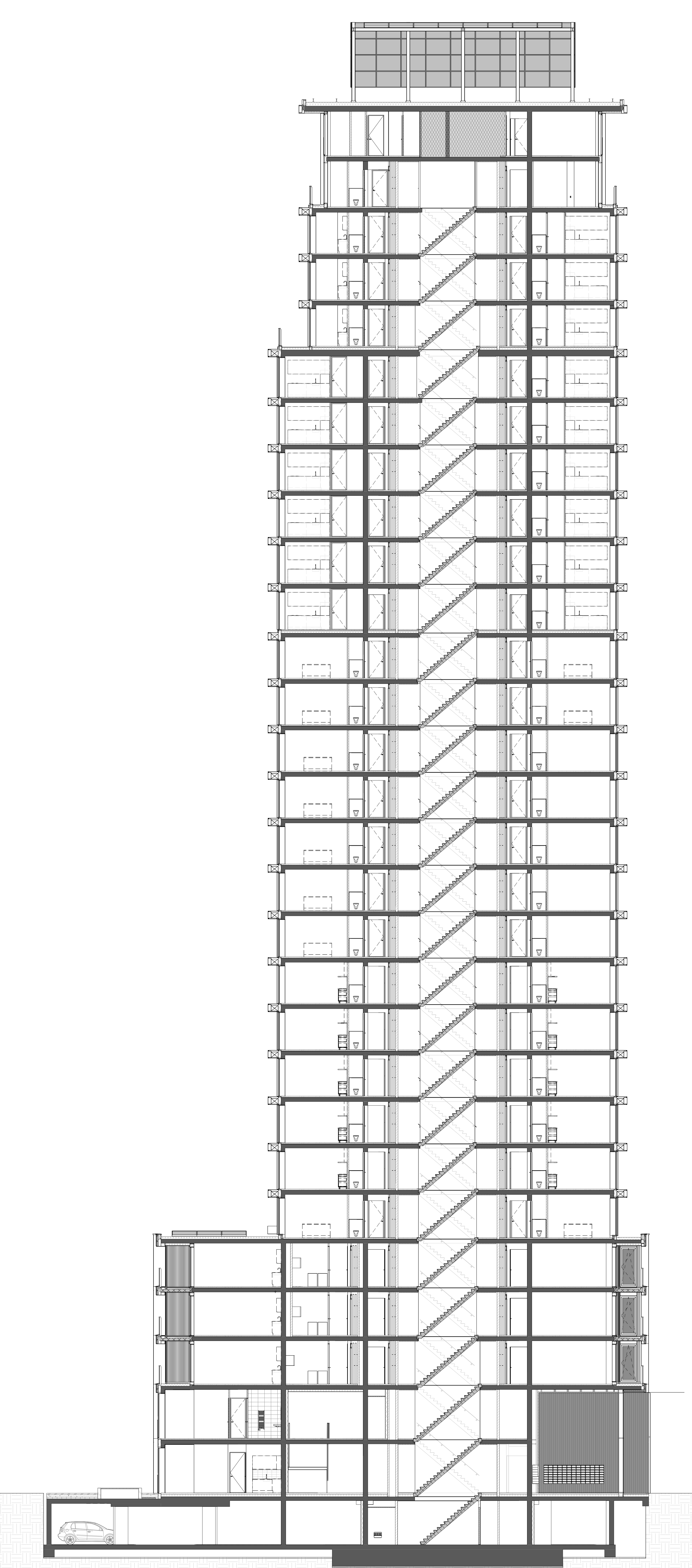
Doorsnede, 1:100
