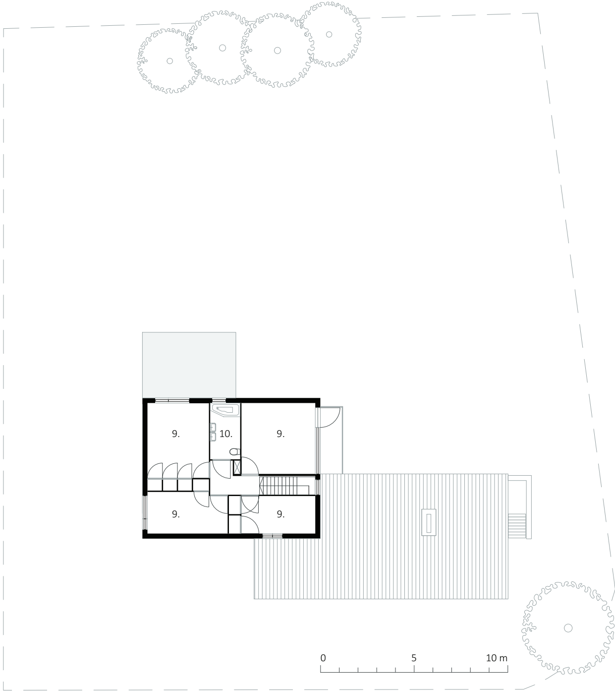
1e verdieping 1968 | 1:200
