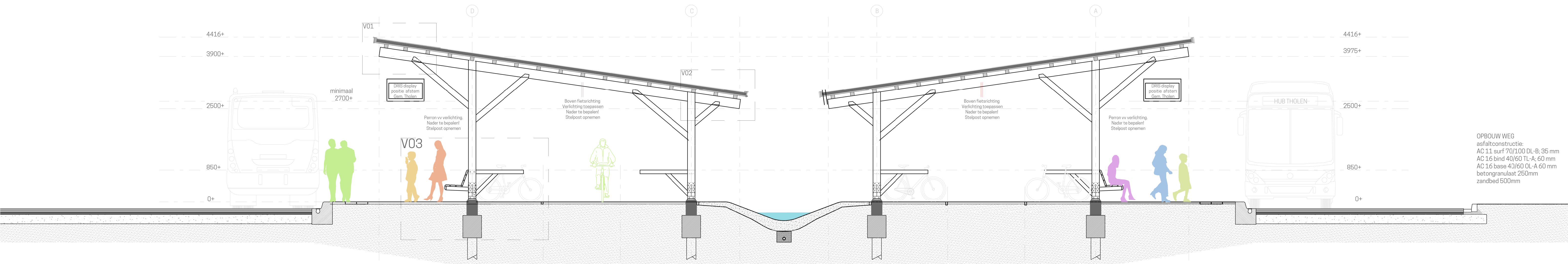
DWARSDOORSNEDE yy' 1-50
