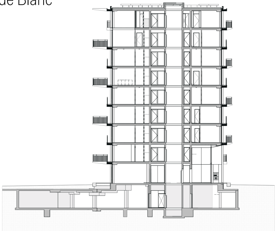
doorsnede Blanc
