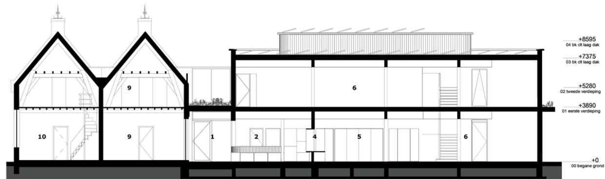
principe doorsnede
