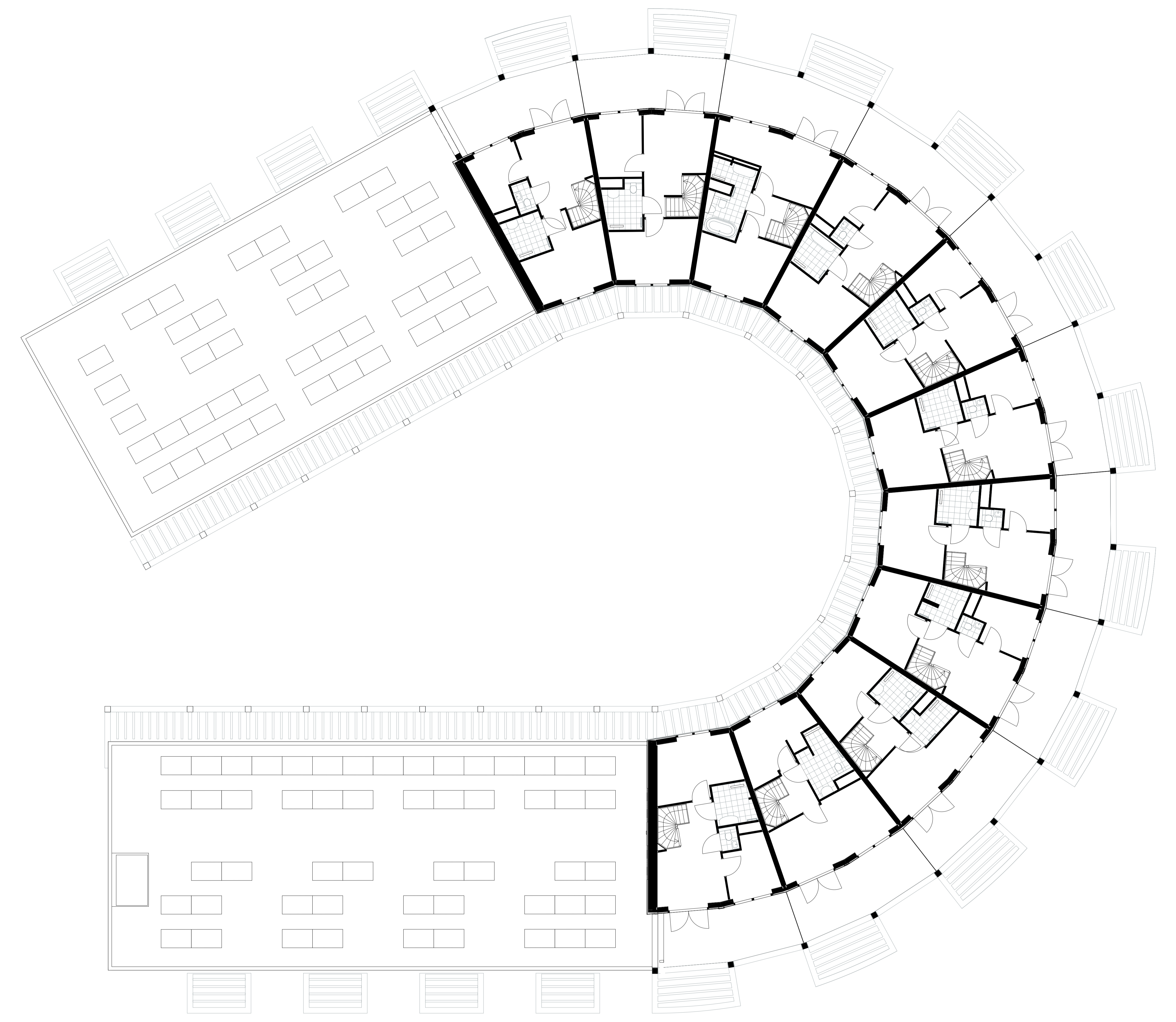
3e verdieping
