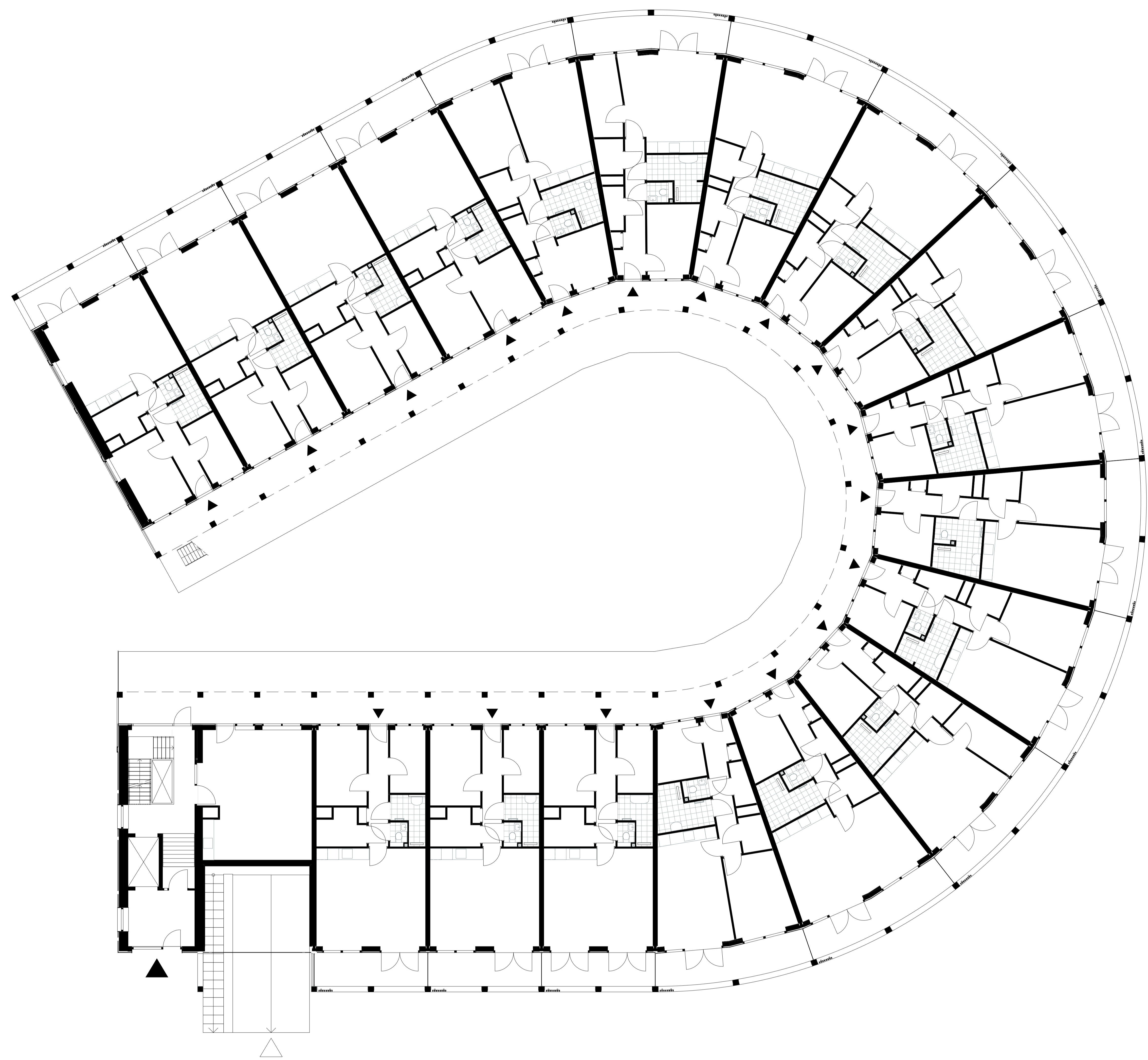
Begane grond
