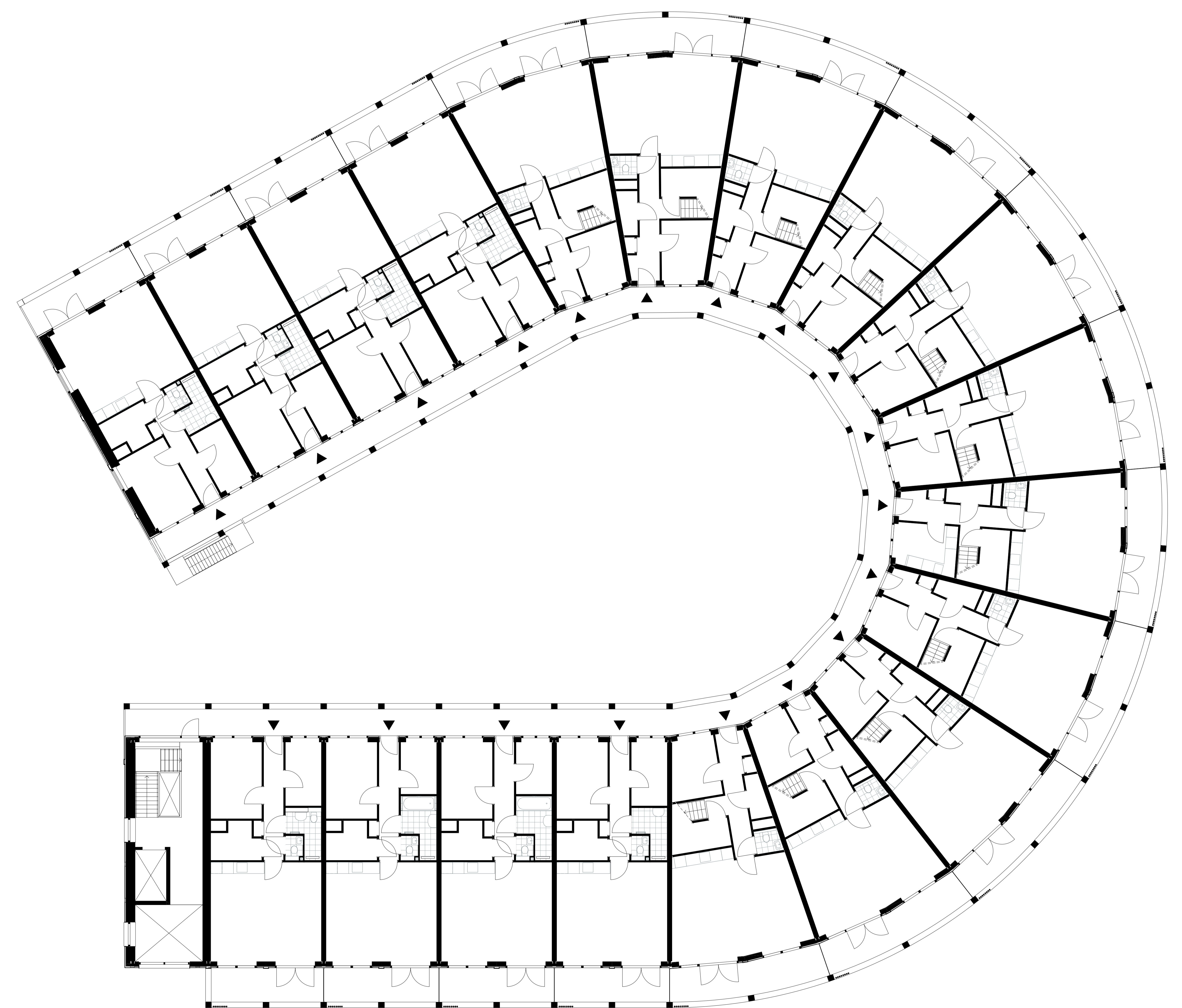
3e verdieping
