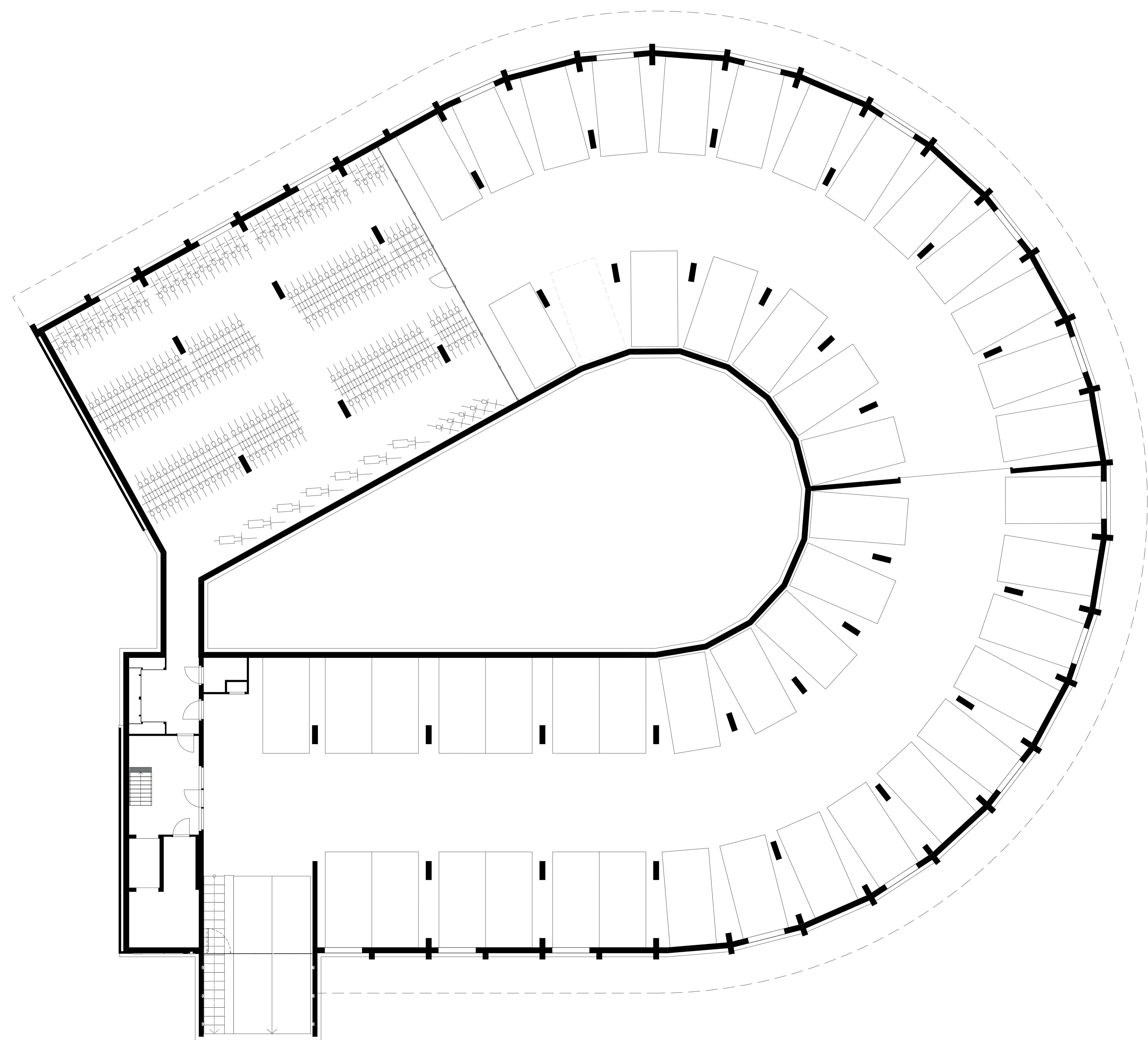
Kelder
