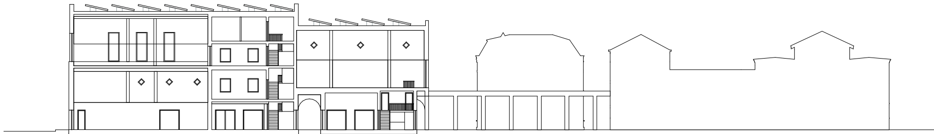
Doorsnede 1:500
