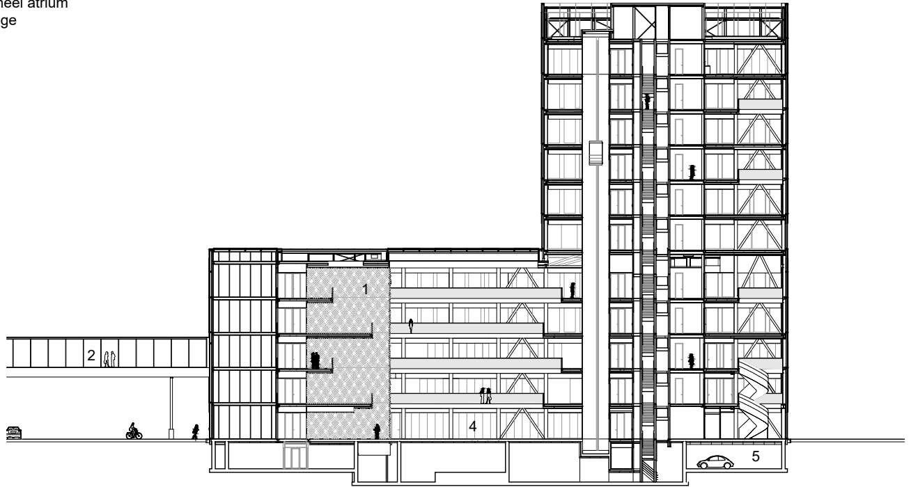
langsdoorsnede
