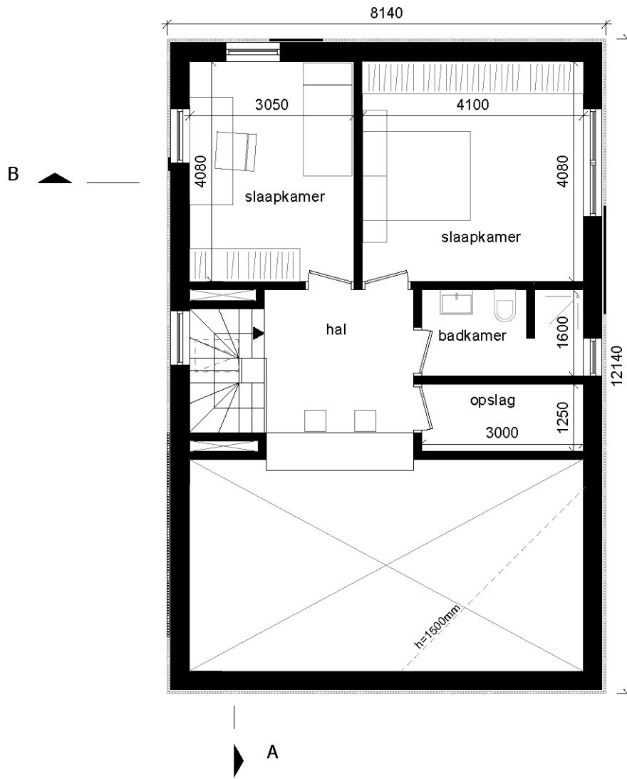
02 eerste verdieping 1 : 100
