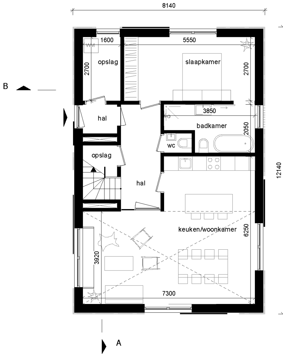
01 begane grond 1 : 100
