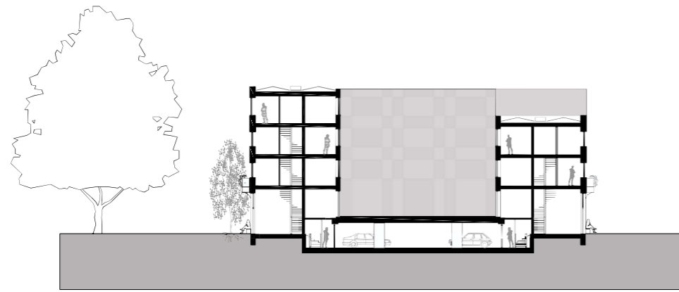
Doorsnede A-A
