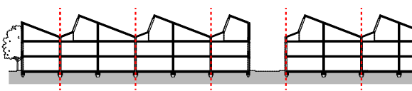
betonnen scheidingswanden zijn uitgezet op een stramienmaat van 7,5 meter, direct afgeleid van de breedtemaat van de oude hallen
