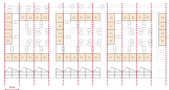
betonconstructie in het zicht op basis van stramien Philips fabriekshallen
