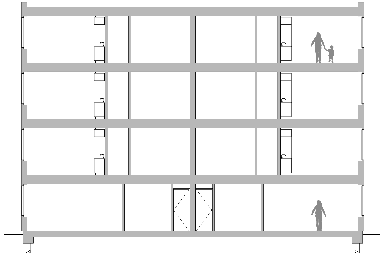
LANGSDOORSNEDE
