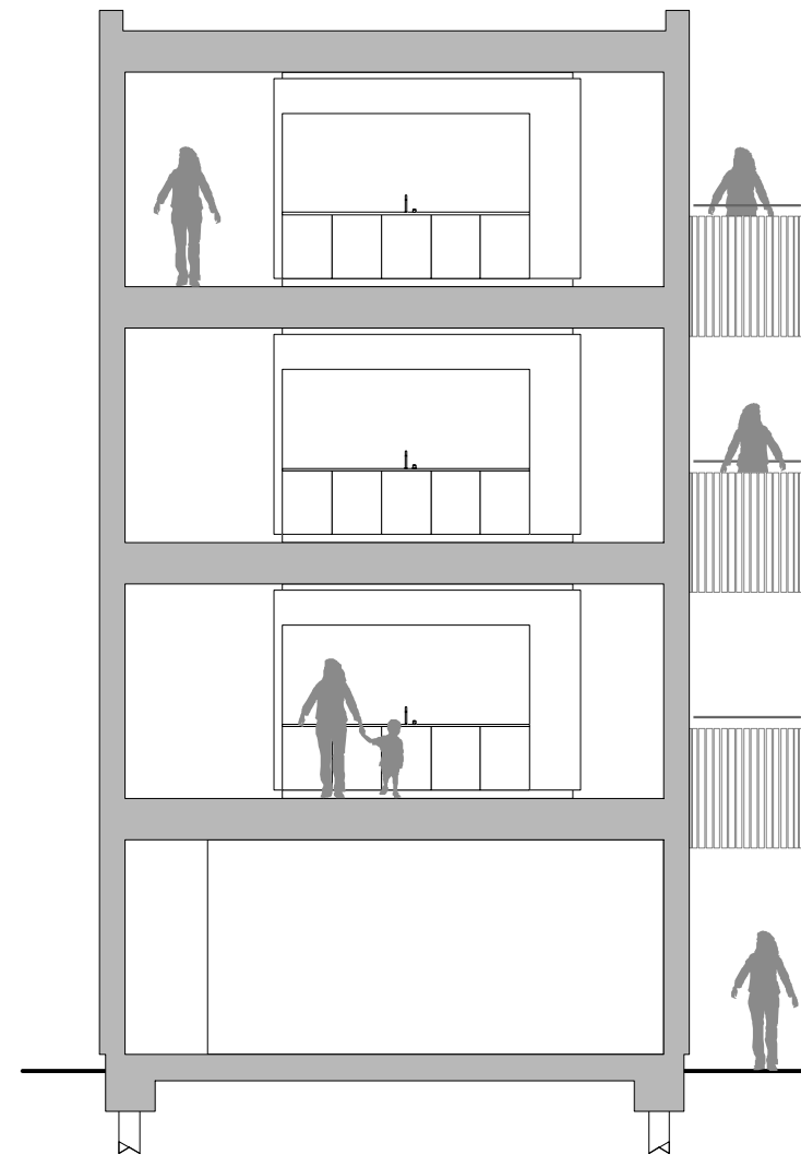
DWARSDOORSNEDE
