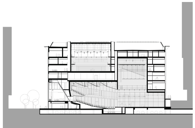
Doorsnede over Danstheaterzaal en Conservatoriumzaal
