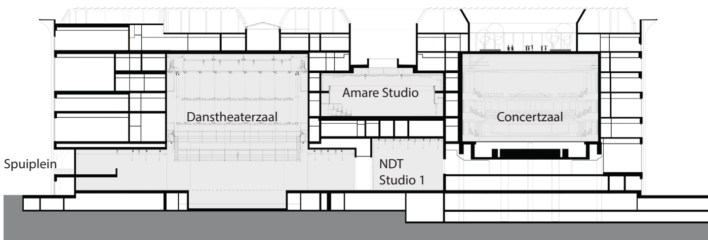
Langsdoorsnede
