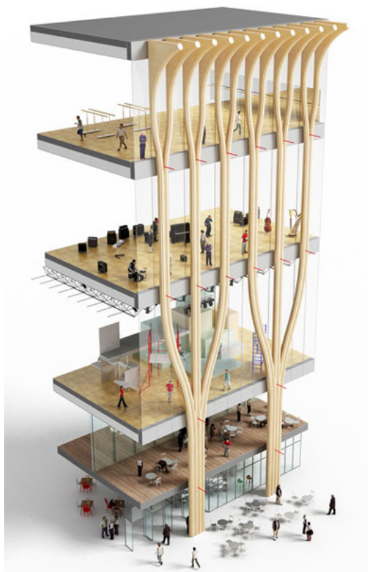
Fragment gevelontwerp
