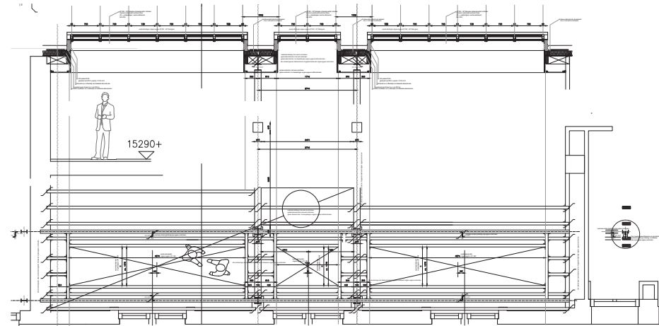
Langsdoorsnede lichtstraat Longitudinal section
