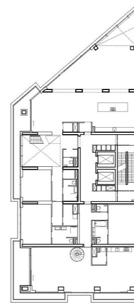
Twintigste verdieping: twee appartementen met twee verdiepingen
