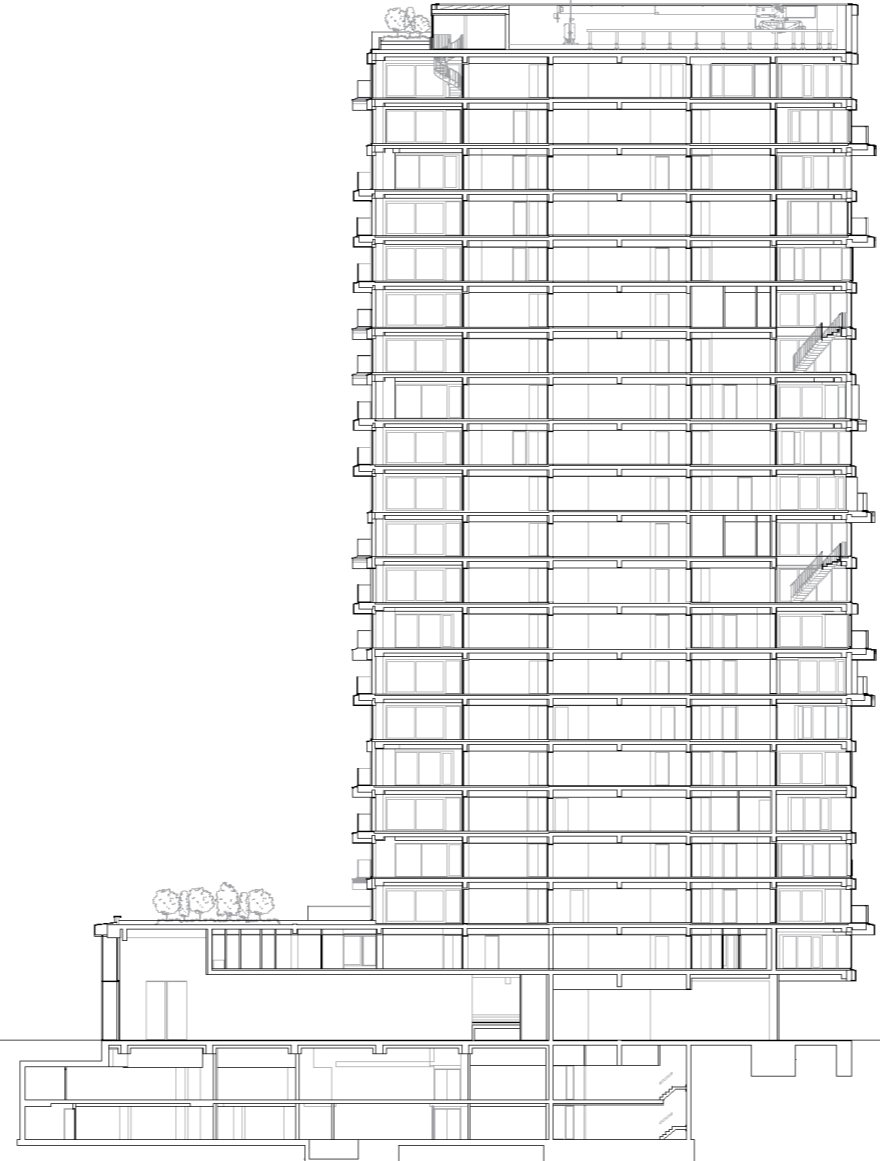
Dwarsdoorsnede
