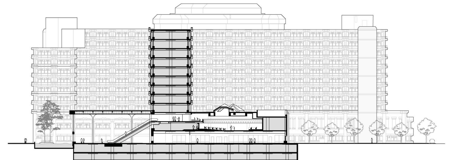
Doorsnede
