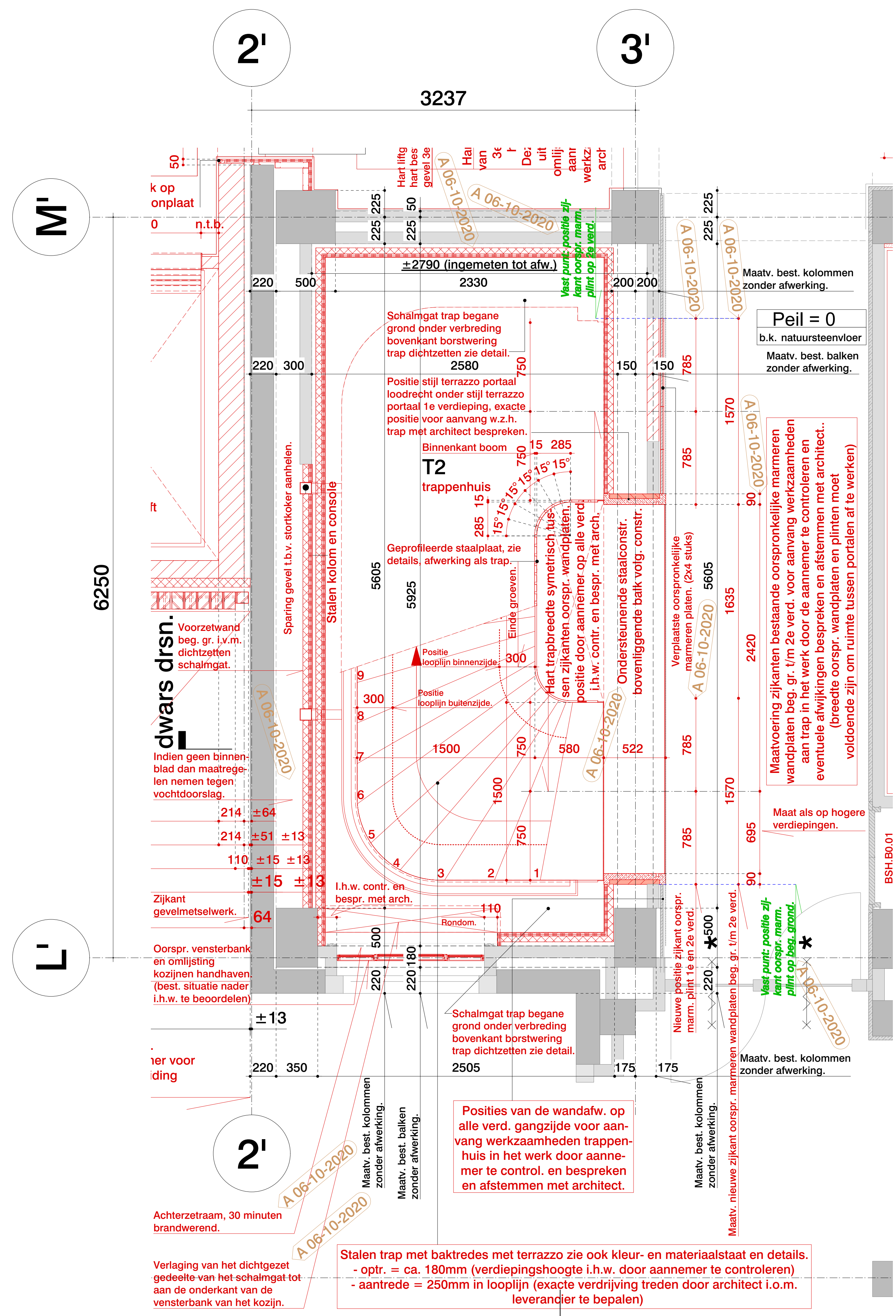
langs drsn. Begane grond
