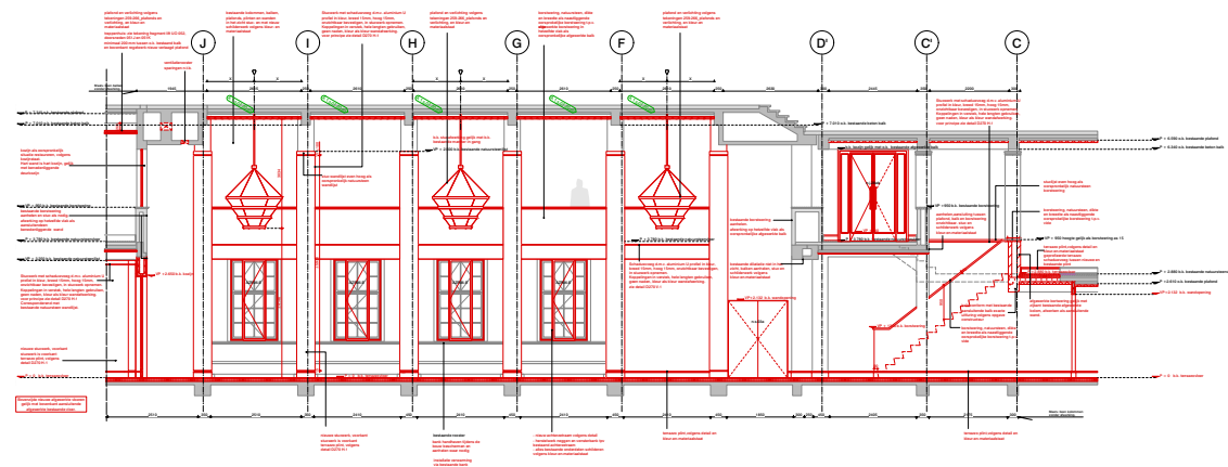
Doorsnede stadsfoyer
