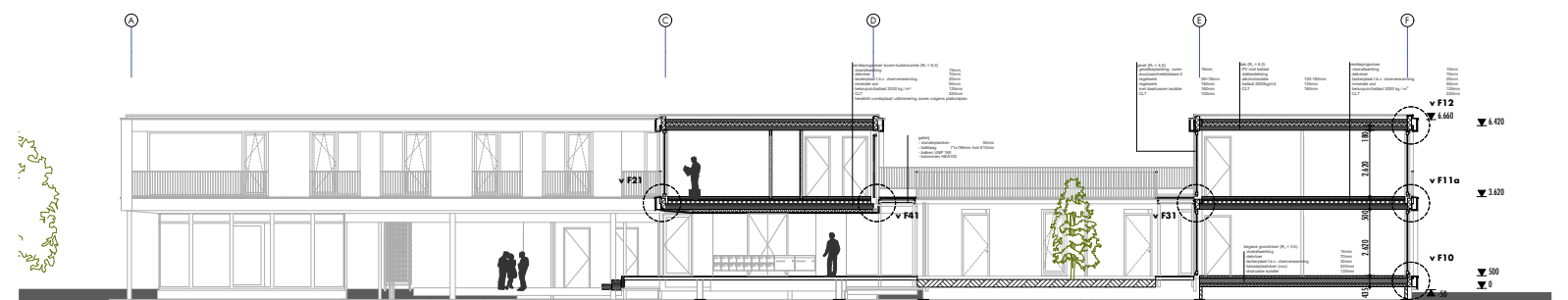
doorsnede FF
