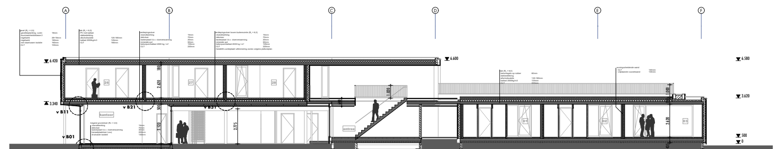
doorsnede BB
