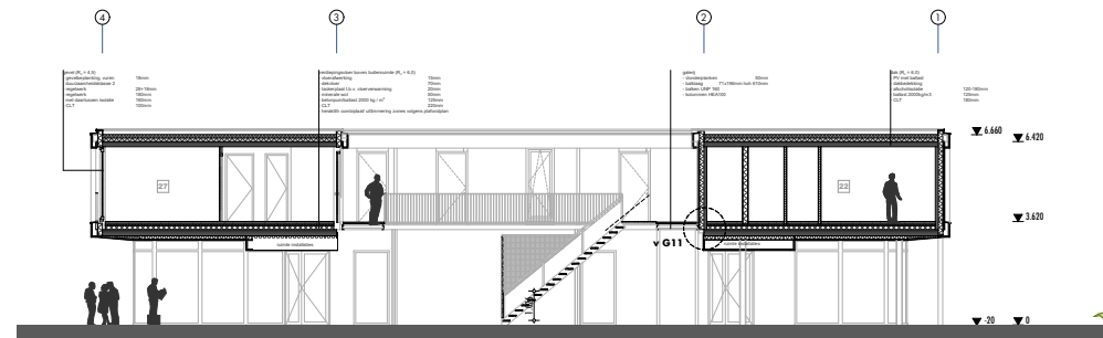
doorsnede GG
