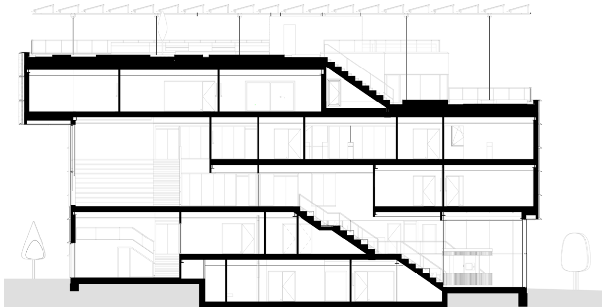
Doorsnede
