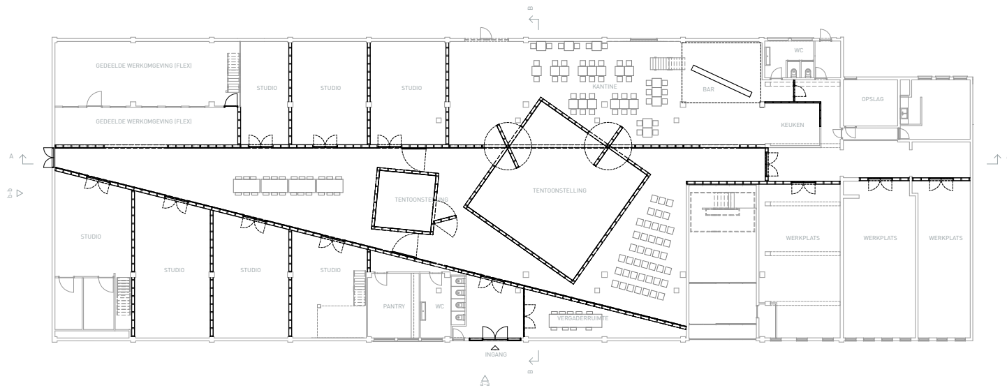
plattegrond
