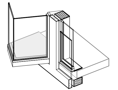
detail 371-309 formaat A2
