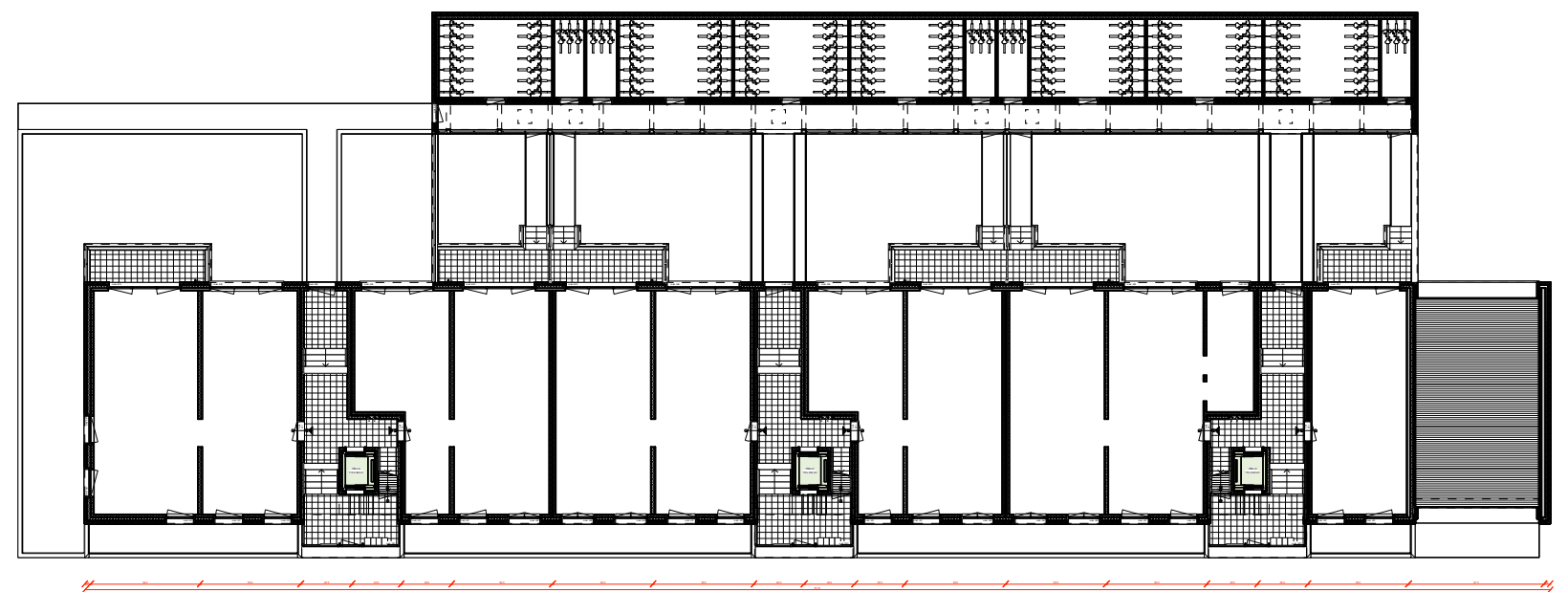
Blok 4, structuur casco gelijkvloers
