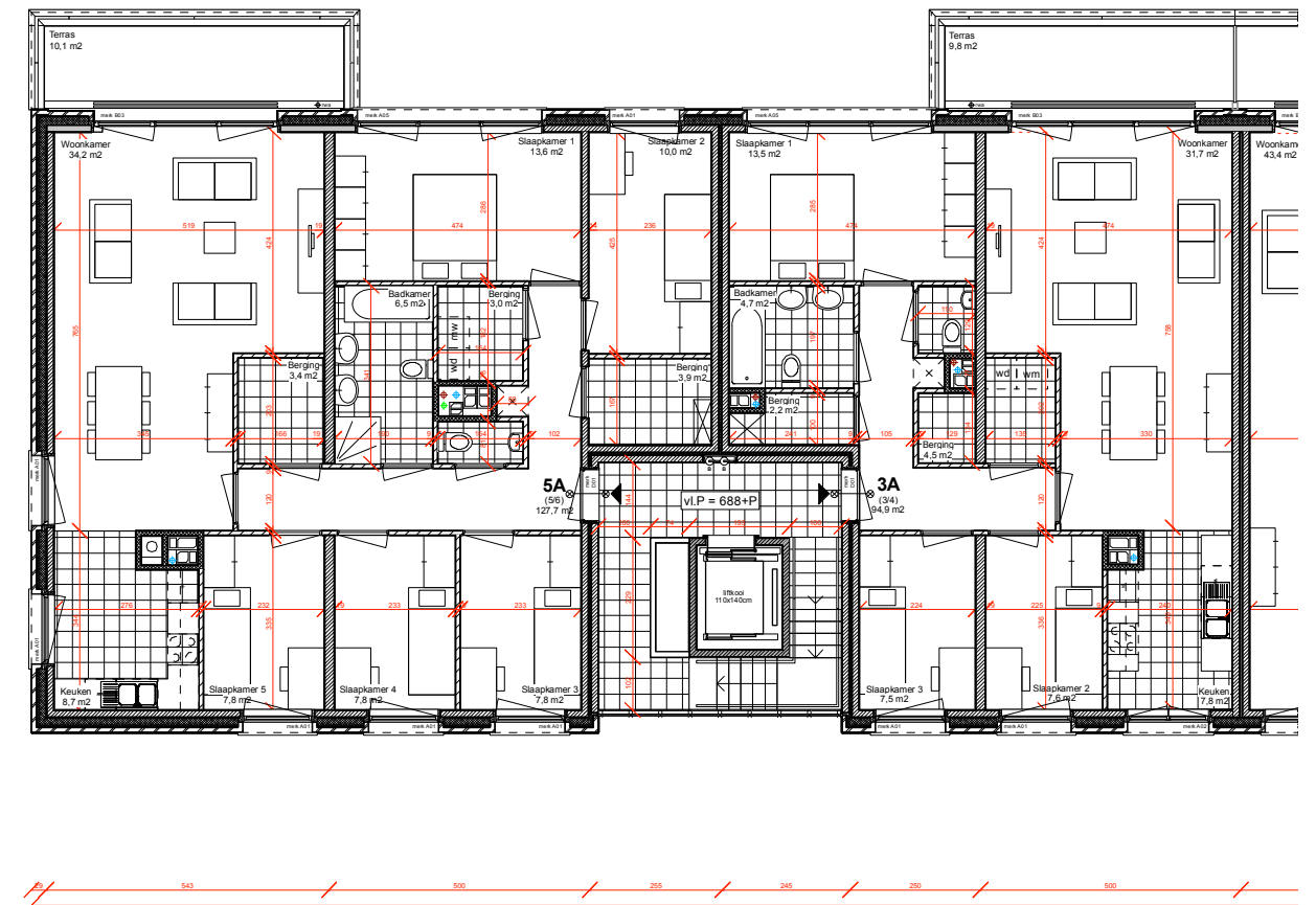
Blok 4, woningverdeling 3 en 4 slaapkamertypes
