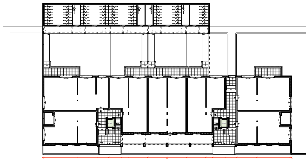
Blok 3, structuur casco gelijkvloers
