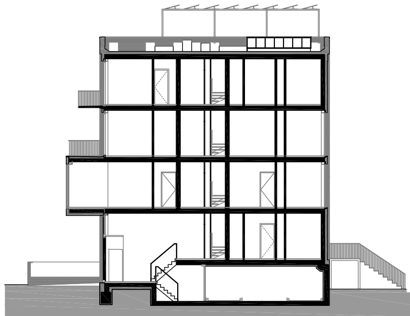
Doorsnede - AA
