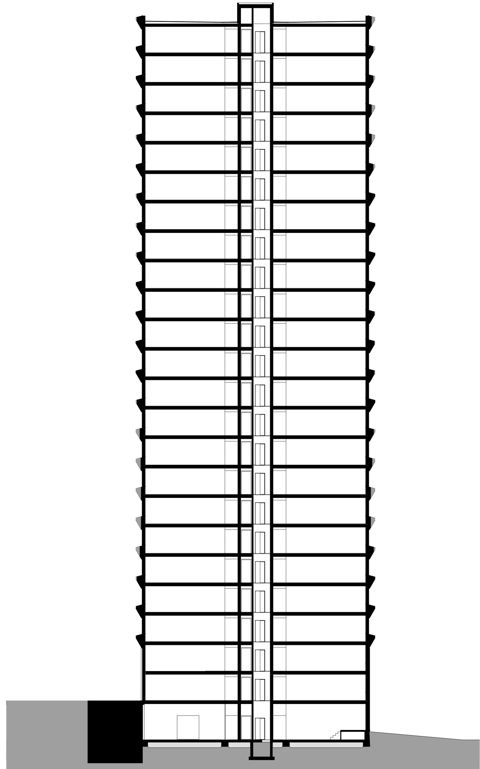
Doorsnede B-B
