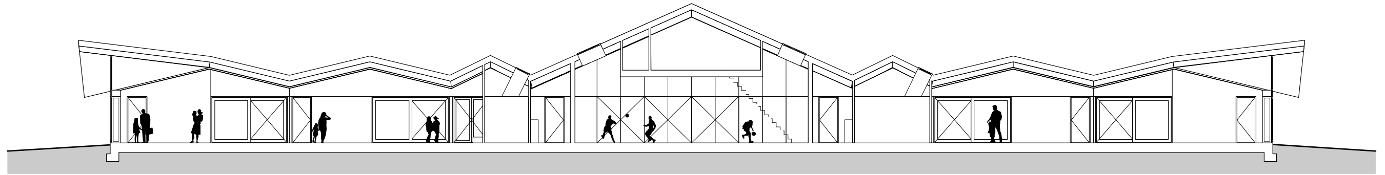
Doorsnede Aa
