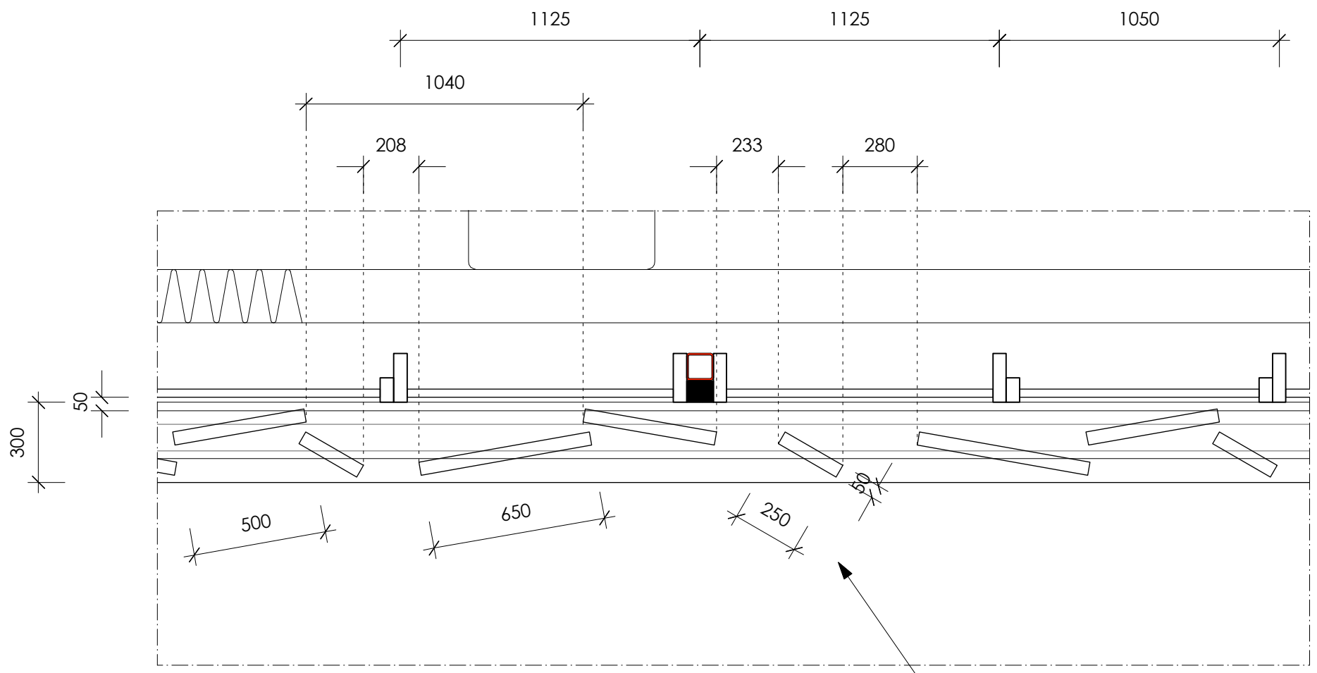
horizontale doorsnede
