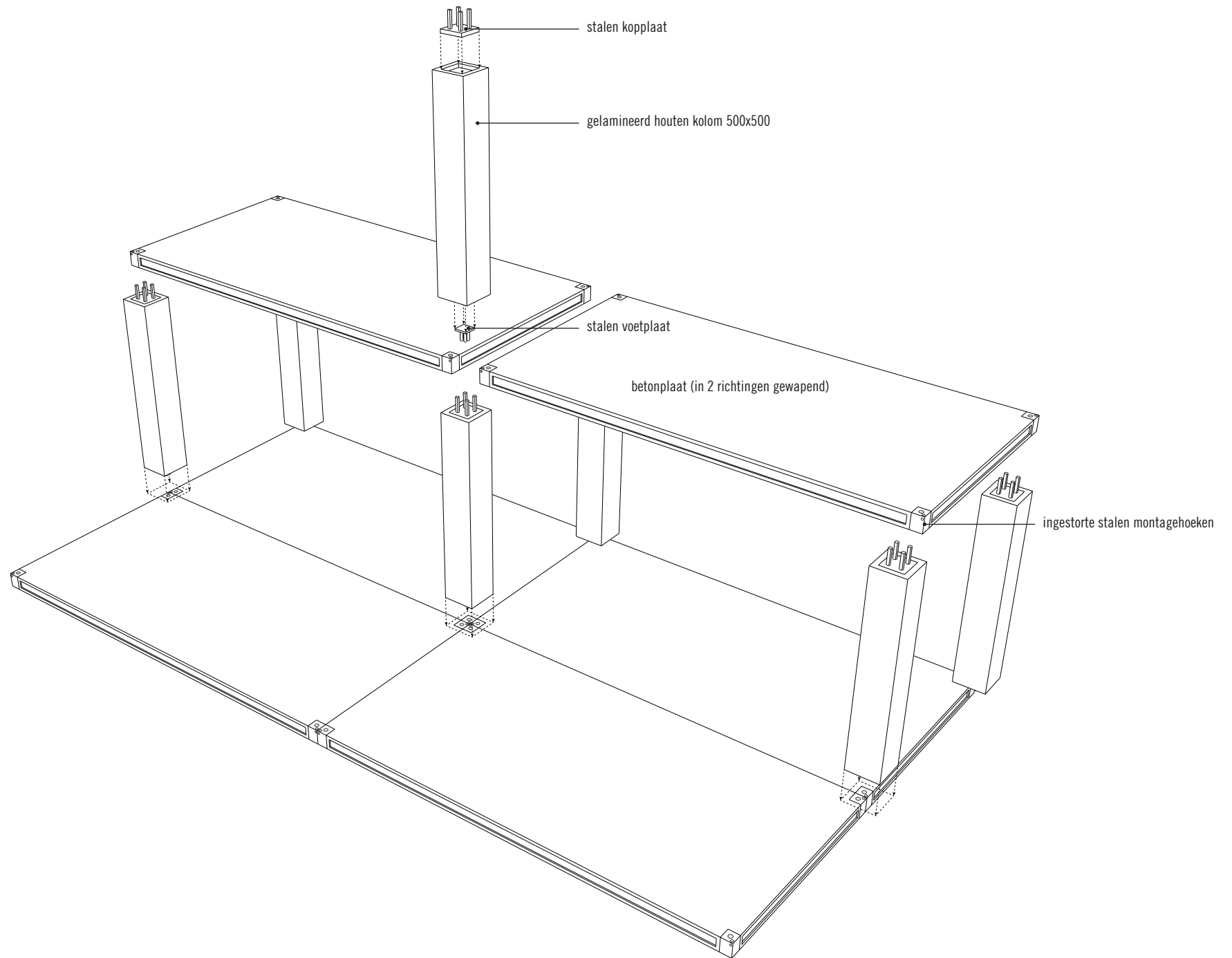
constructie & montageprincipe CD20 systeem met houten kolommen
