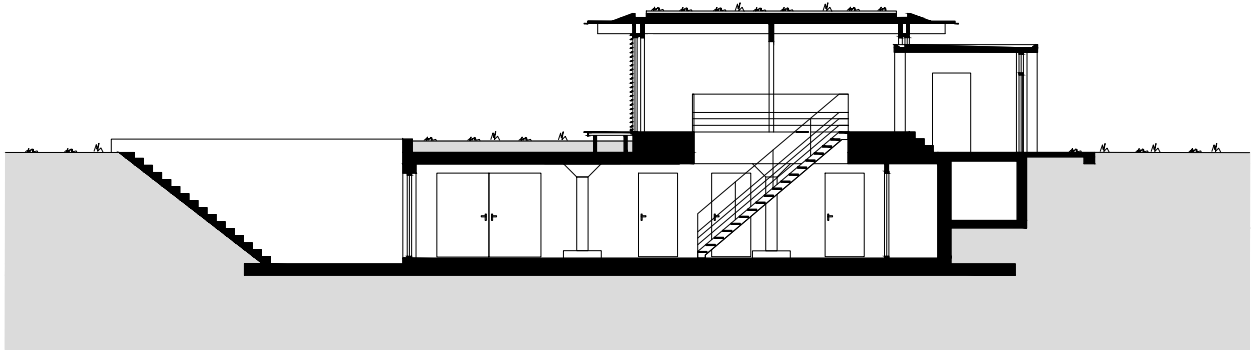
Langsdoorsnede A-A
