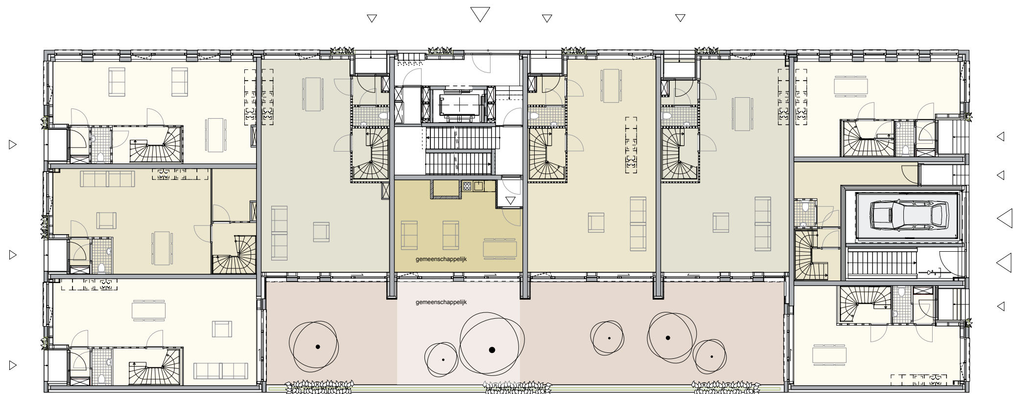
begane grond
