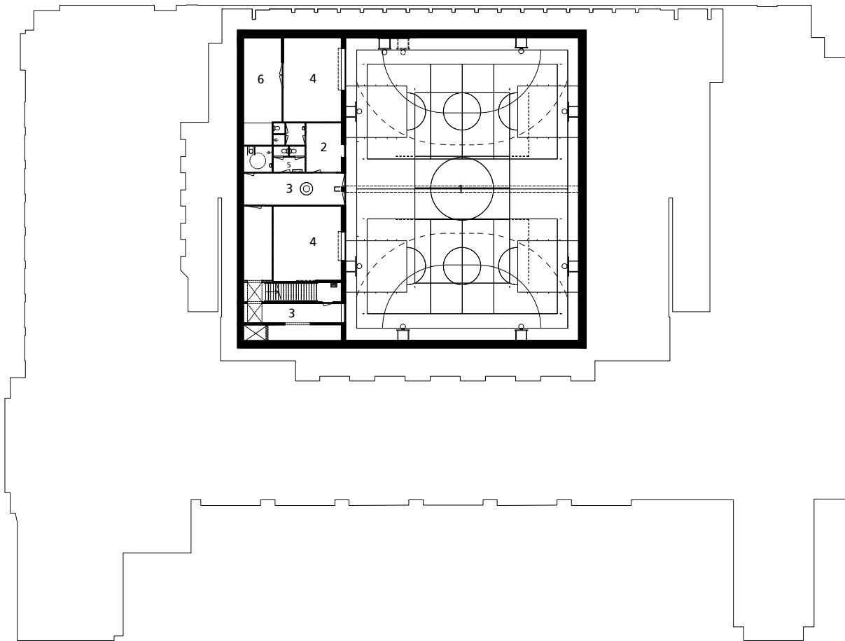
plattegrond verdieping -3 nieuwe situatie 9364-P
