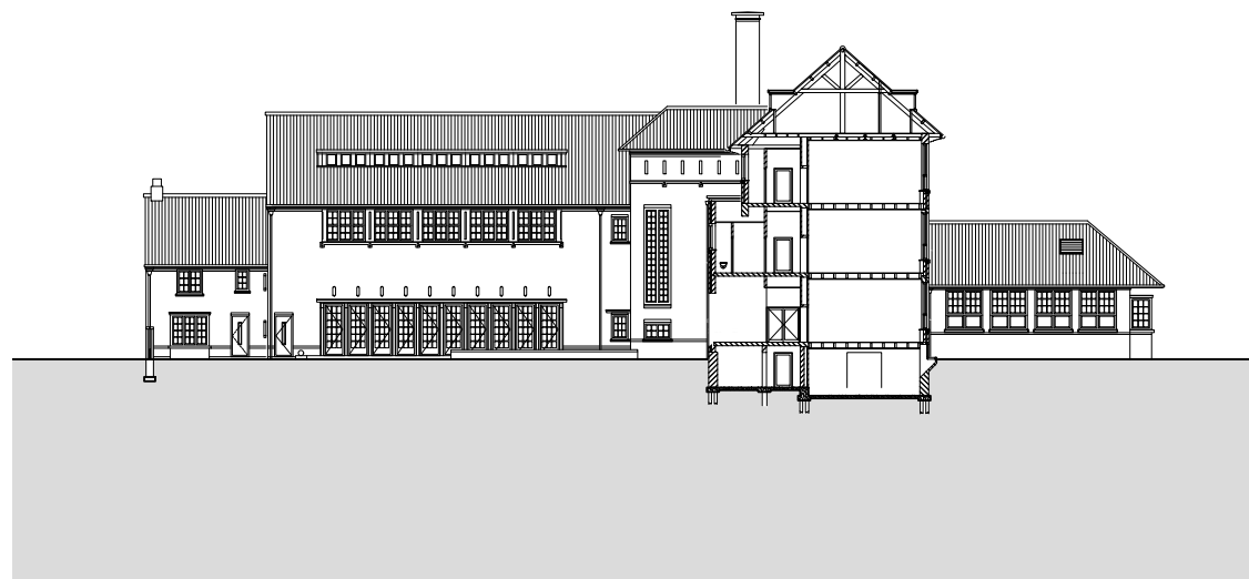
doorsnede B-B bestaande situatie
