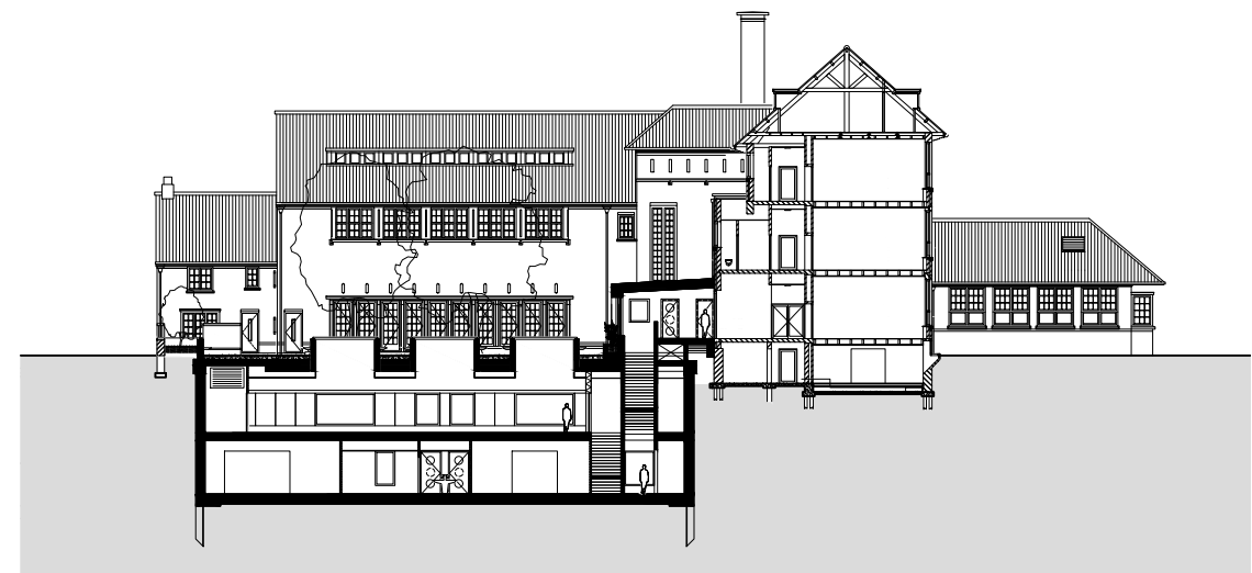
doorsnede B-B nieuwe situatie
