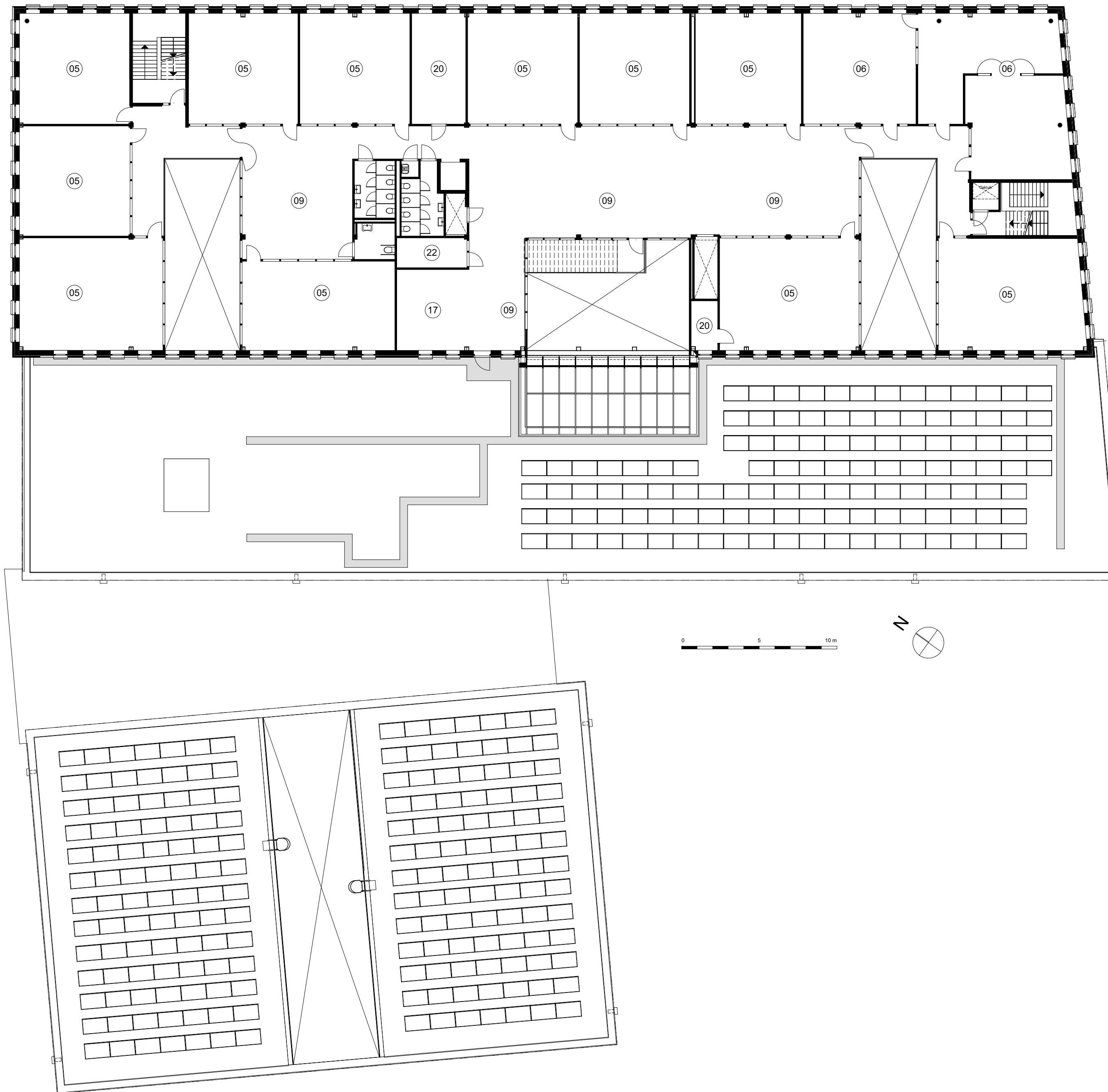
Plattegrond 2de verdieping
