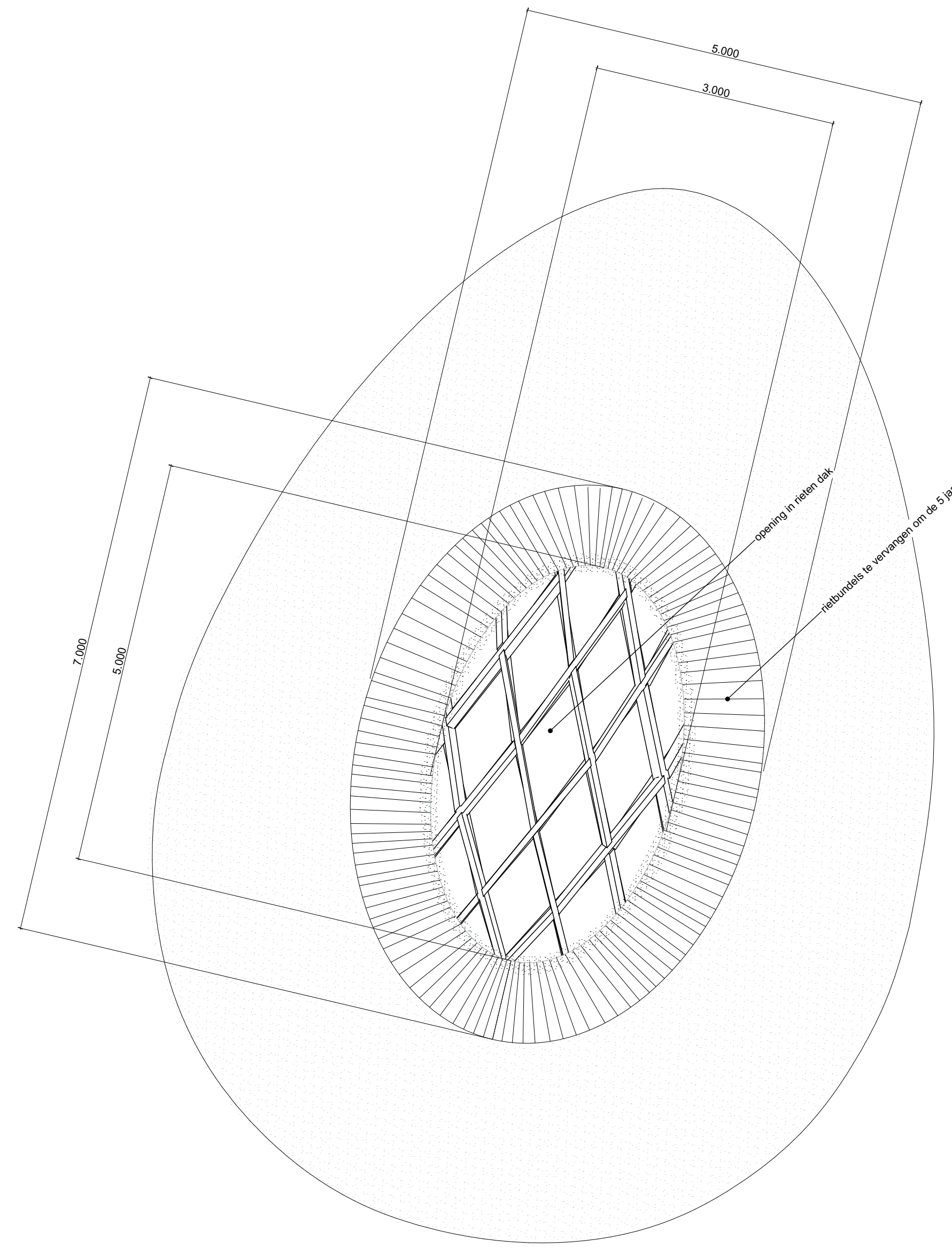
Bovenaanzicht
