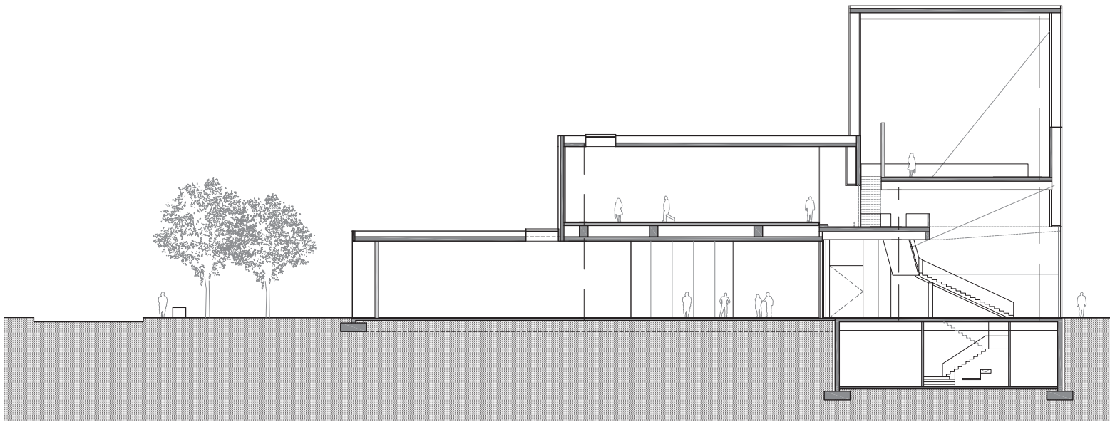
Sectio c-c'
