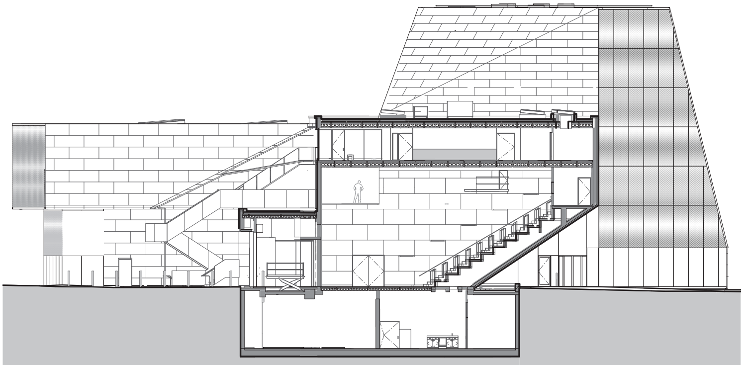
Sectio b-b'
