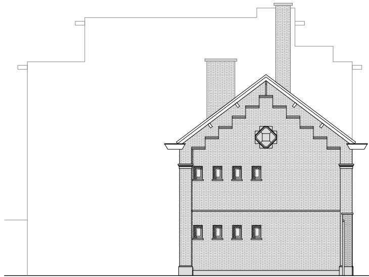
zijgevel bestaand
