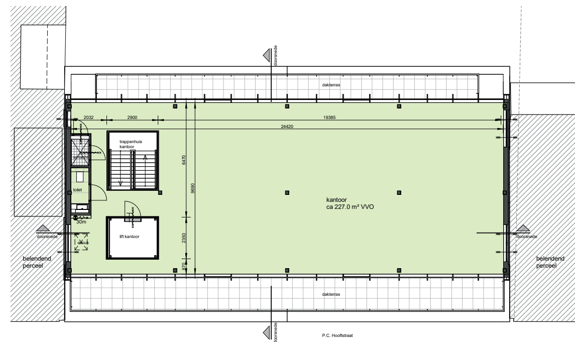
4e verdieping
