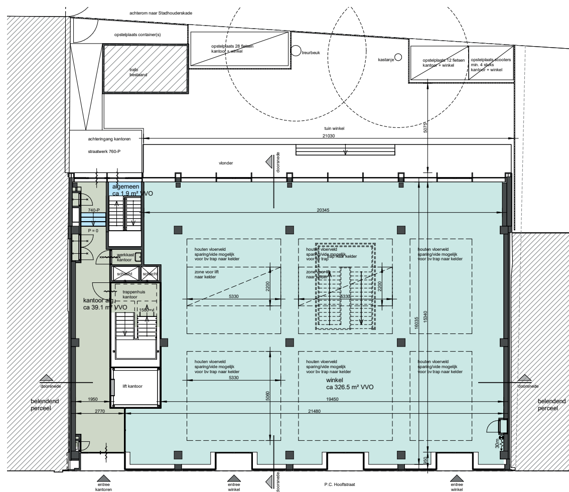
Begane grond
