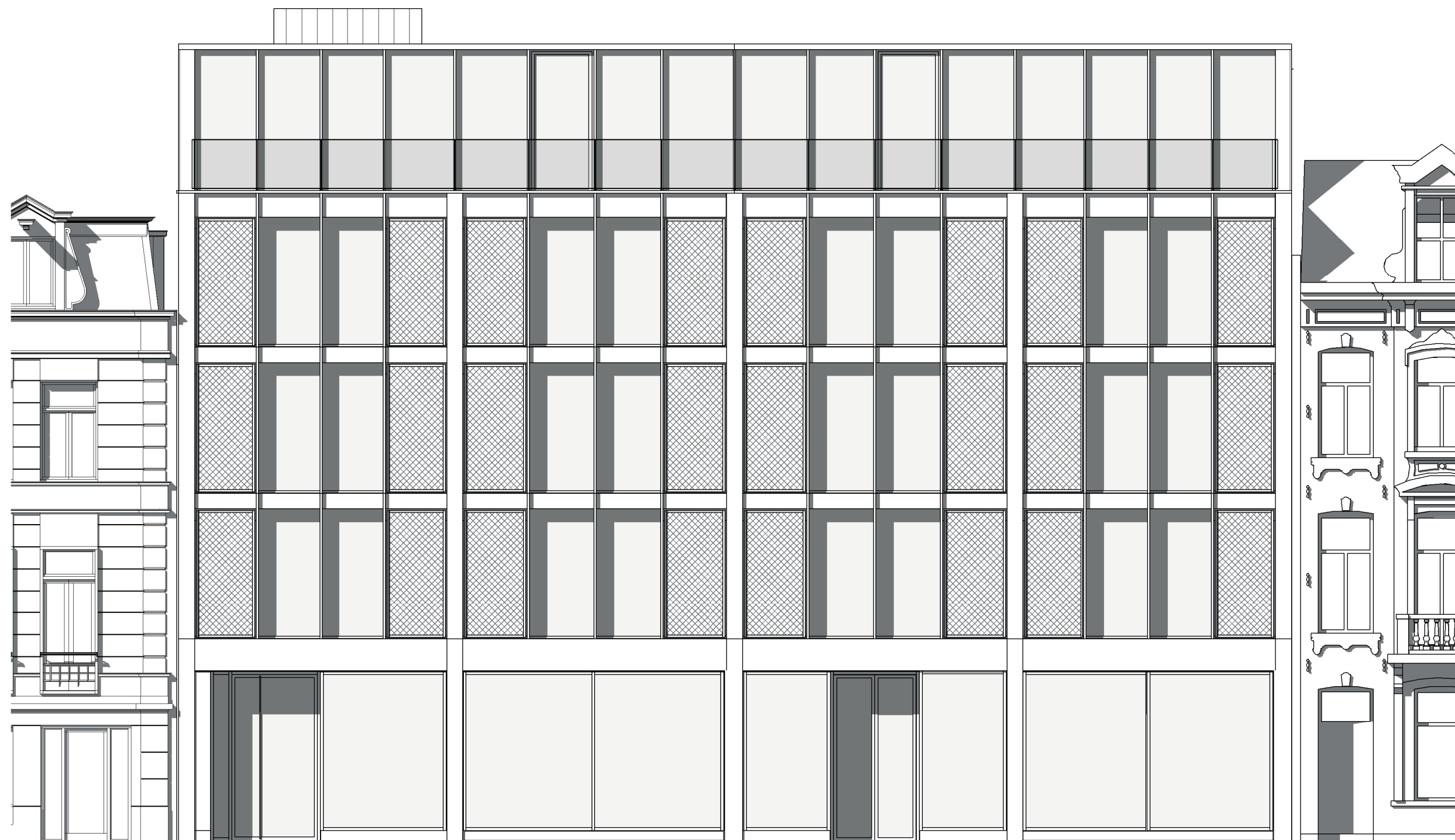
Straatgevel
