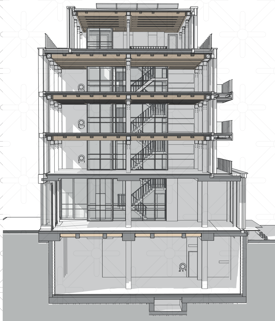
Dwarsdoorsnede
