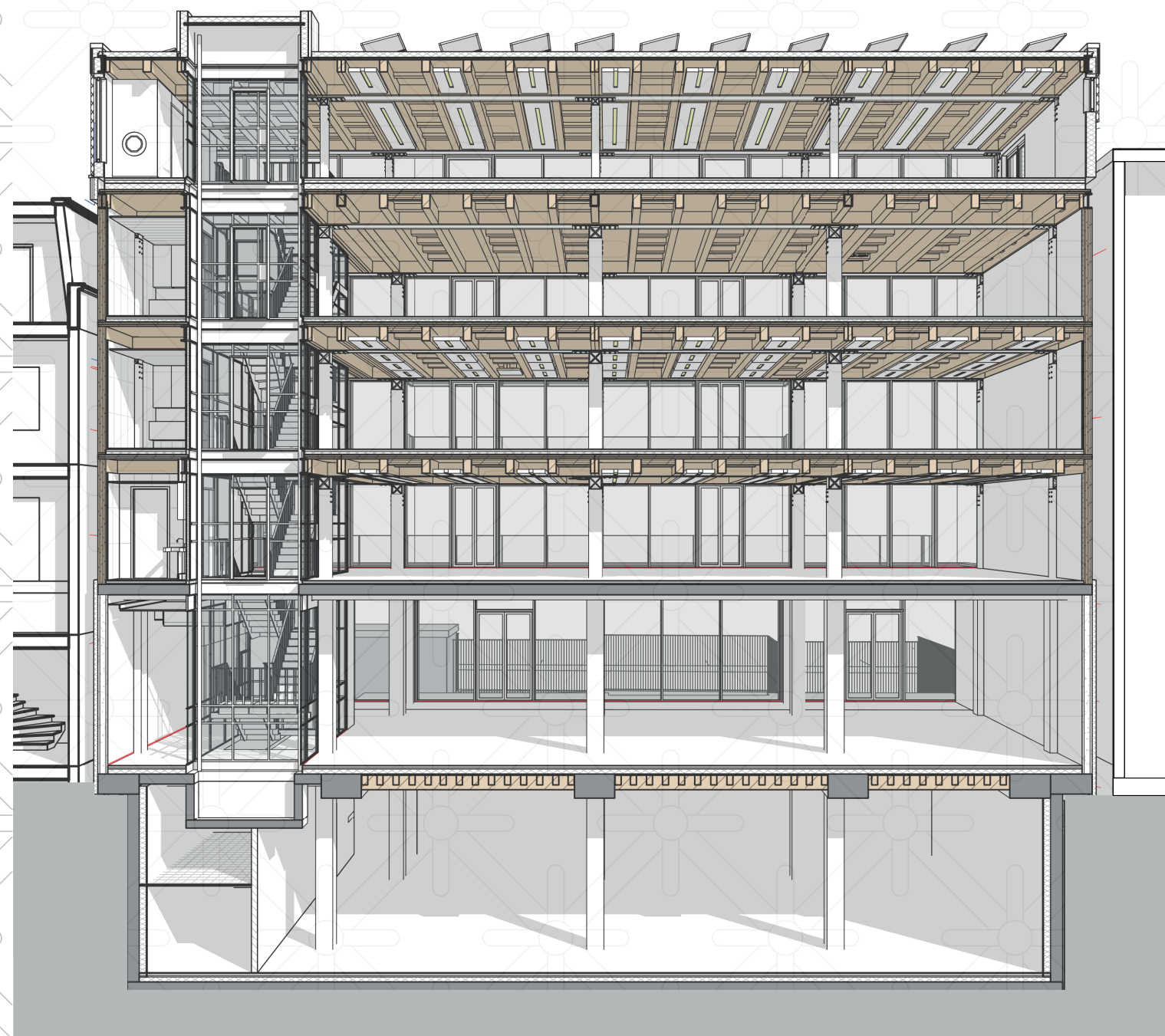
Langsdoorsnede
