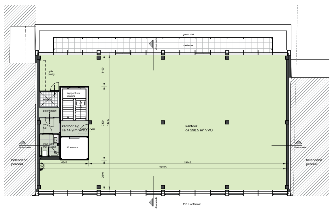
1e t/m 3e verdieping
