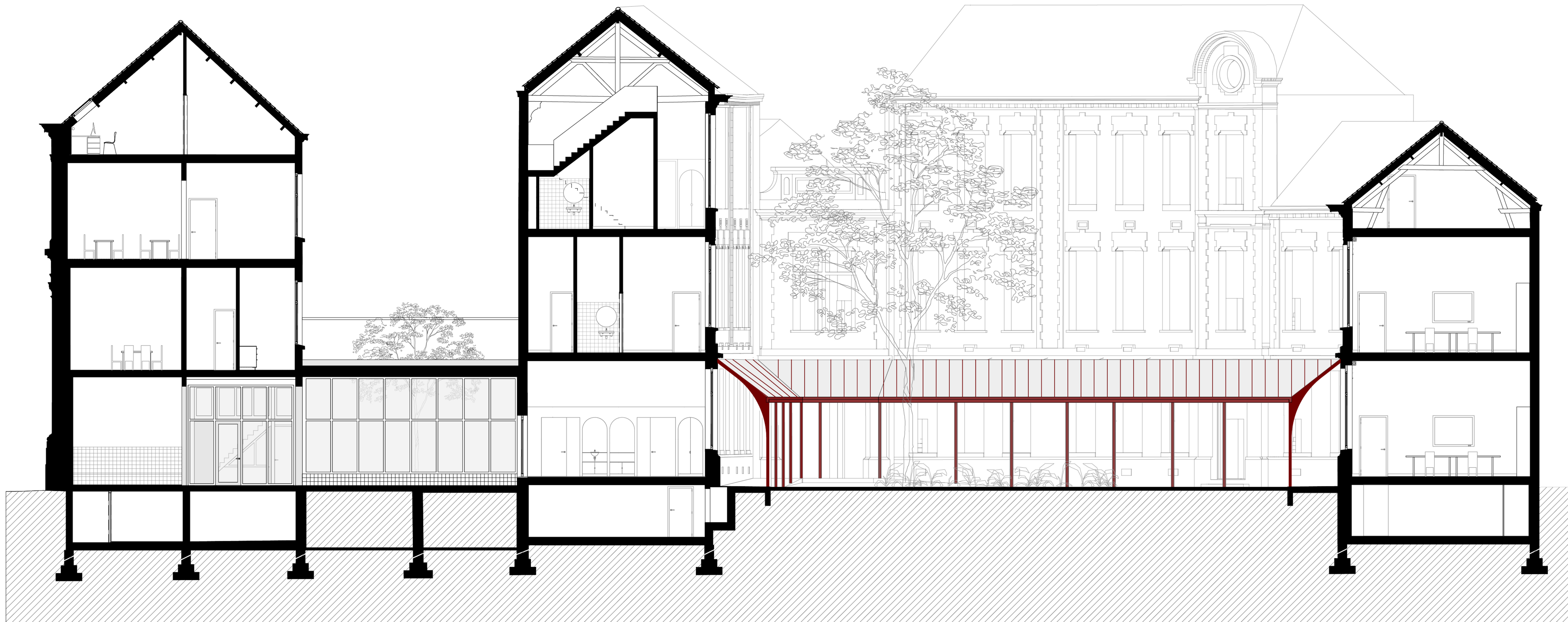
snede AA'
