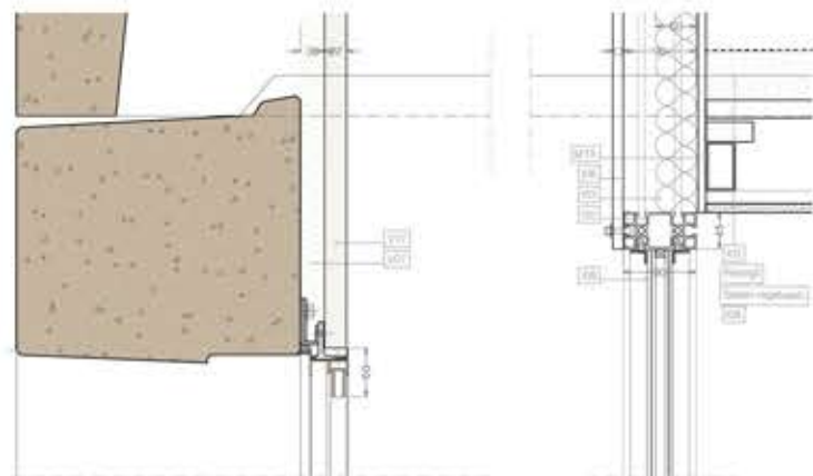
Snede Detail 1 - 1/5
