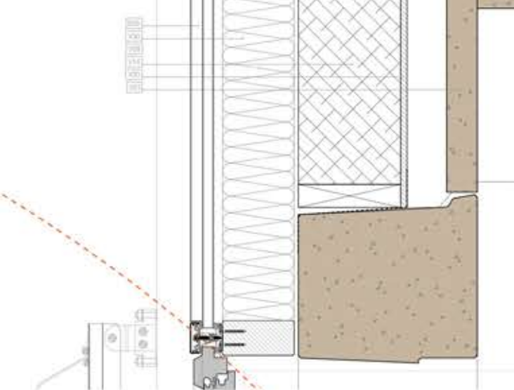
Snede Detail 2 - 1/5
