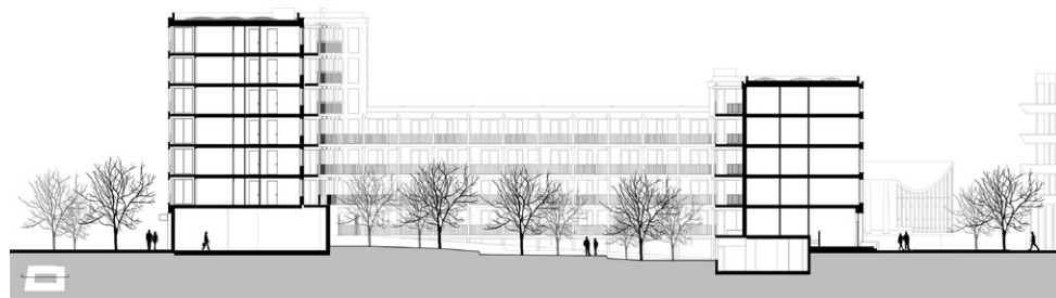
Dwarsdoorsnede
