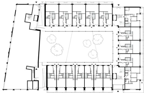
Begane grond
