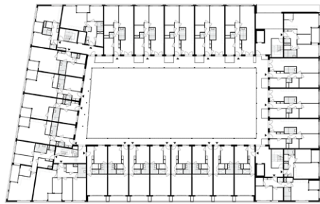
1 e verdieping
