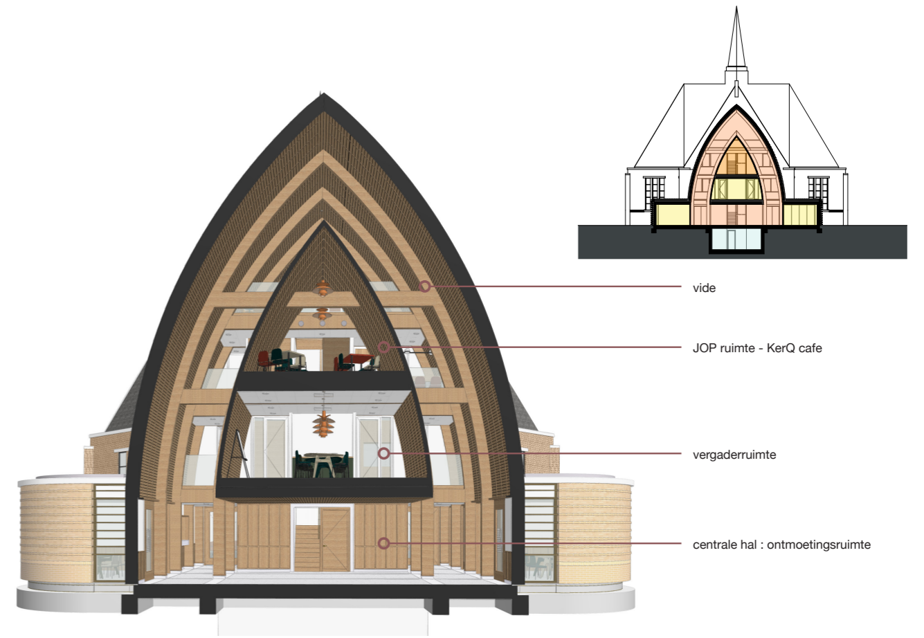
Dwarsdoorsnede
