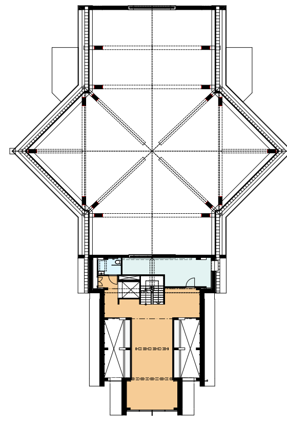
Tweede verdieping | plattegrond
