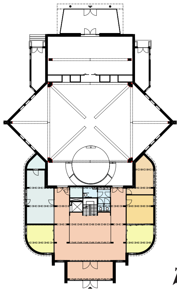
Begane grond | plattegrond
